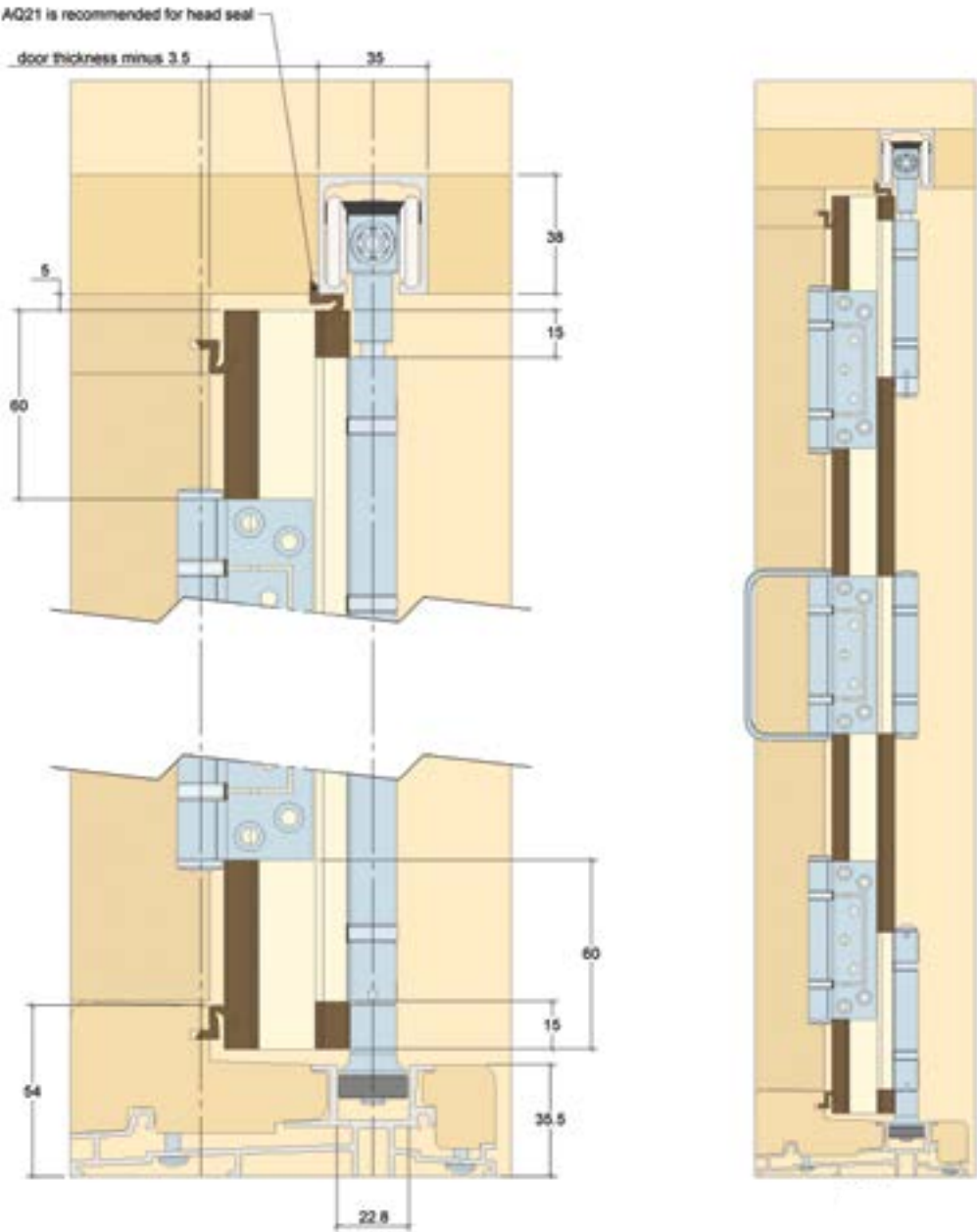
E2-004.DXF
